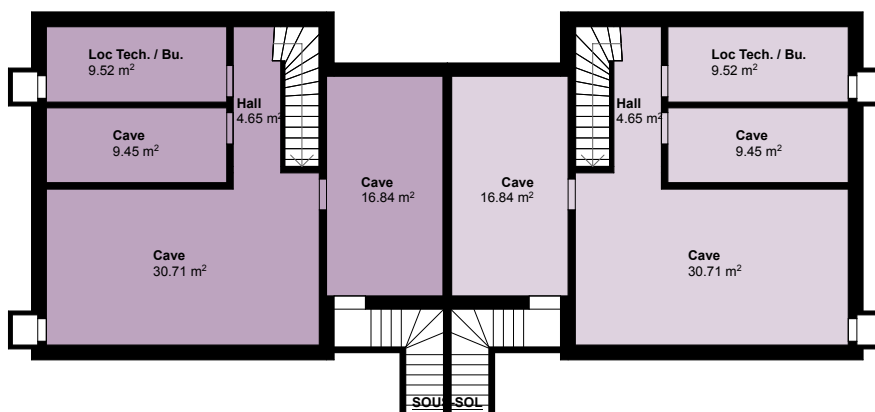
SOUS-SOL
